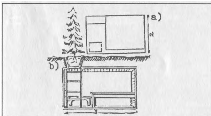
Jono Žemaičio bunkeris : a) planas, b) skersinis pjūvis. įėjimas į bunkerį maskuojamas eglute.
