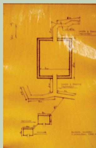
Buvusio Kauno bunkerio planas (sudarė ir braižė V. Striužas).
