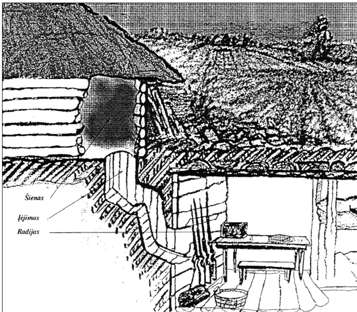
87. „Tauro“ apygardos „Geležinio vilko“ rinktinės štabo bunkeris (Piešinys iš KGB archyvų). Tomo Kajacko rekonstrukcija.
