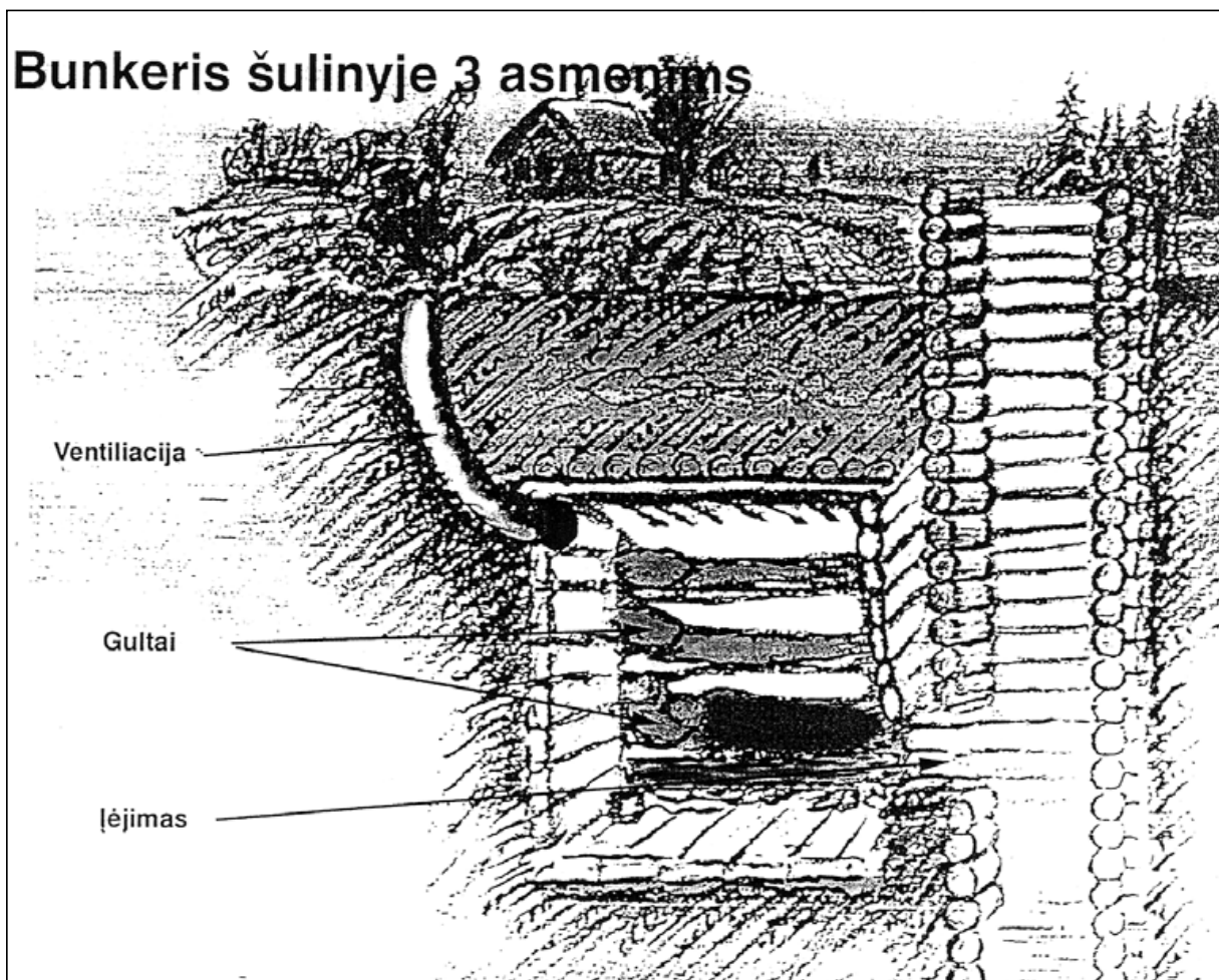
86. Bunkeriš šulinyje 3 asmenims (Piešinys iš KGB archyvų). Tomo Kajacko rekonstrukcija.
