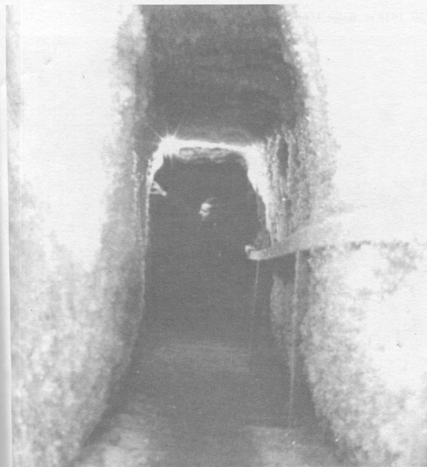
16. Įšalą tyrinėjanti laboratorija
