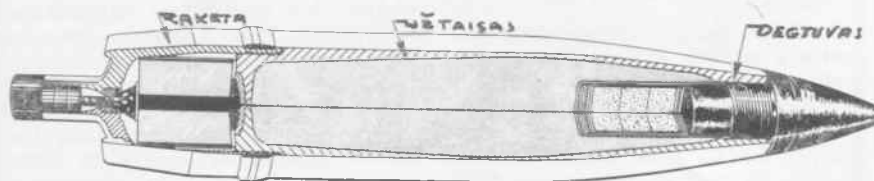
105 mm pabūklų sviedinio raketa veikia 1.8 sekundės, po 23 sekundžių palikus vamzdį.
